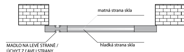
posuvné křídlo pravé (posuv doprava) / Pravé posuvné křídlo (posouváné doprava)
