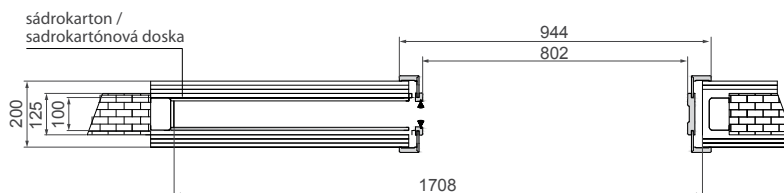
Zárubeň rozsah / Záruben rozsah (126-200) – SYMETRICKÁ*
