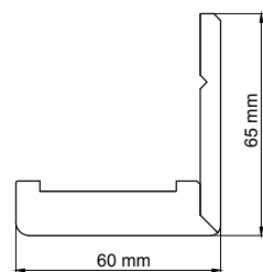
Rozšiřující Záklop pro nastavitelnou zárubeň - šířka 60 mm / Rozšiřující záklop pre nastaviteľnú obložku - šířka 60 mm
