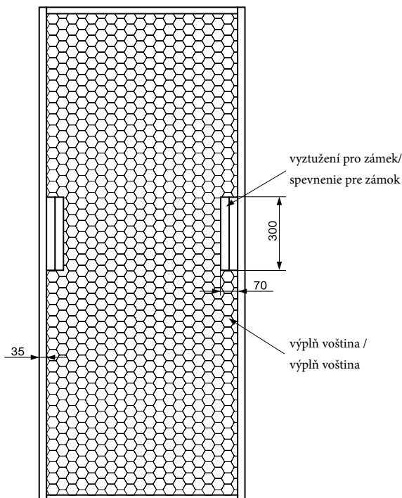
Konstrukce deskového křídla / Konštrukcia doskového křídla
