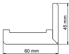
Záklop pro nastavitelnou zárubeň - šířka 60 mm / Záklop pre nastaviteľnú obložku - šířka 60 mm
