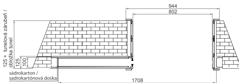
Zárubeň rozsah / Záruben rozsah (200-220) DO (400-420) – ASYMETRICKÁ
