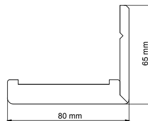
Rozšiřující Záklop pro nastavitelnou zárubeň - šířka 80 mm / Rozšiřující záklop pre nastaviteľnú obložku - šířka 80 mm
