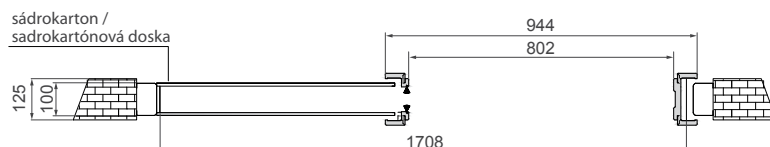
Zárubeň rozsah / Záruben rozsah 125 - PEVNÝ / PEVNÝ
