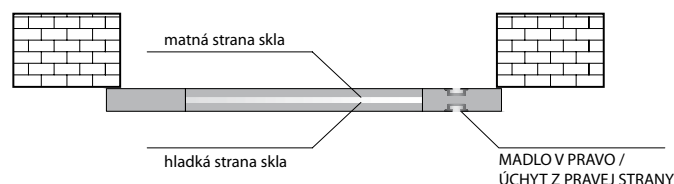
posuvné křídlo pravé (posuv doprava) / Pravé posuvné křídlo (posouváné doprava)
