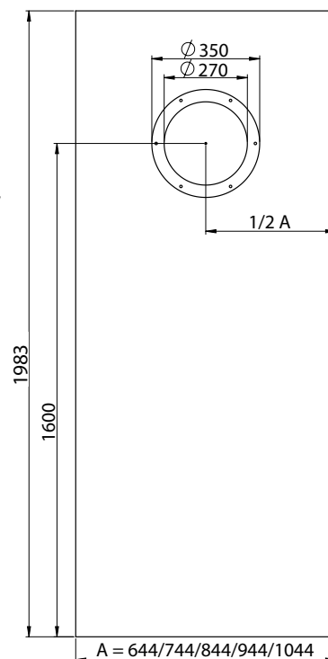
Konstrukce křídla Bulaj / Konštrukcia křídla Bulaj
