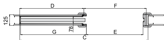
Jednodílné stavební pouzdro G/K dveřní křídlo / Jednodielna kazeta G/K dveřné křídlo
