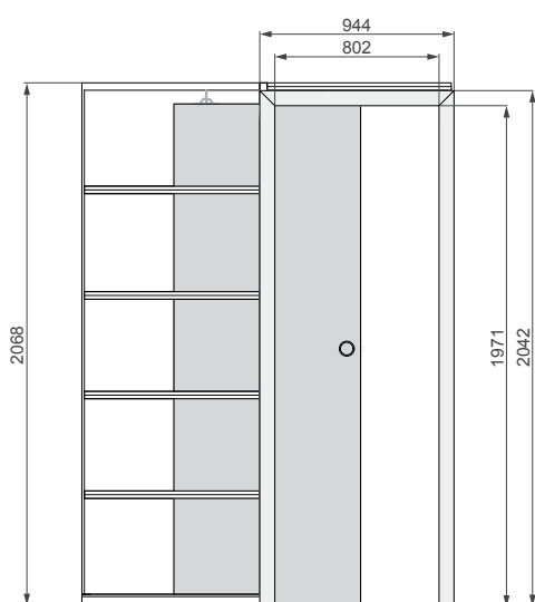
Zárubeň rozsah / Zárubňa rozsah (200-220) DO (400-420) – ASYMETRICKÁ
