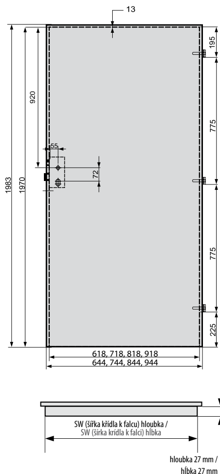
FALCOVÉ KŘÍDLO V CSN STANDARDU / FALCOVÉ KRÍDLO V CSN ŠTANDARDU
