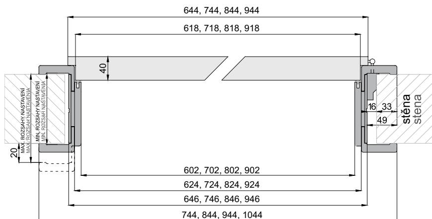
Ostění pro nastavitelnou zárubeň - šířka 80 mm / Ostenie pre nastaviteľnú zárubňu - šířka 80 mm
