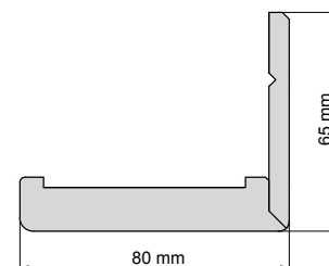
Ostění rozšiřující pro nastavitelnou zárubeň - šířka 80 mm / Ostenie rozširujúci pre nastaviteľnú zárubňu - šířka 80 mm
