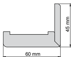
Ostění pro nastavitelnou zárubeň - šířka 60 mm / Ostenie pre nastaviteľnú zárubňu - šířka 60 mm
