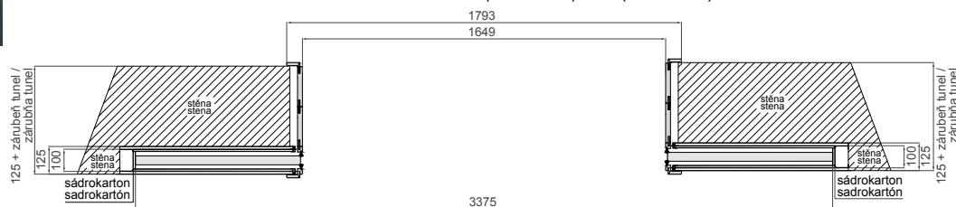
ZÁRUBEŇ ROZSAH / ZÁRUBŇA ROZSAH (200-220) DO (400-420) - ASYMETRICKÁ
