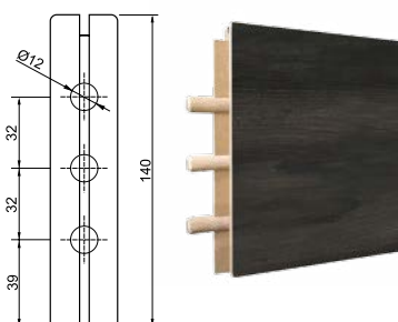
DOLNÍ RÁM CSN STANDARD / DOLNÝ RÁM CSN STANDARD
