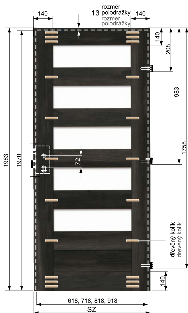
FALCOVÉ KŘÍDLA V CSN STANDARDU / FALCOVÉ KRÍDLA V CSN ŠTANDARDU
