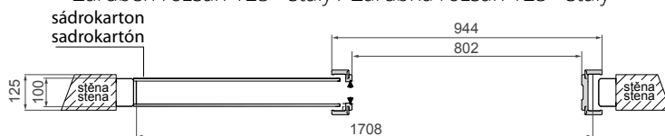
Zárubeň rozsah / Zárubňa rozsah (126-200) – SYMETRICKÁ*
