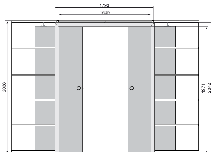
ZÁRUBEŇ ROZSAH 125 - STÁLÝ / ZÁRUBŇA ROZSAH 125 - STÁLÝ
