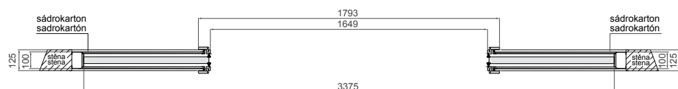
ZÁRUBEŇ ROZSAH 125 - STÁLÝ / ZÁRUBŇA ROZSAH 125 - STÁLÝ
