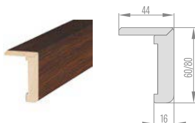
ŠTANDARDNÝ L-PROFIL PRE NASTAVI- TEĽNÉ ZÁRUBNE
