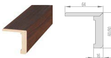
L-PROFIL S PREDĽŽENÝM PEROM PRE NASTAVITEĽNÉ ZÁRUBNE
